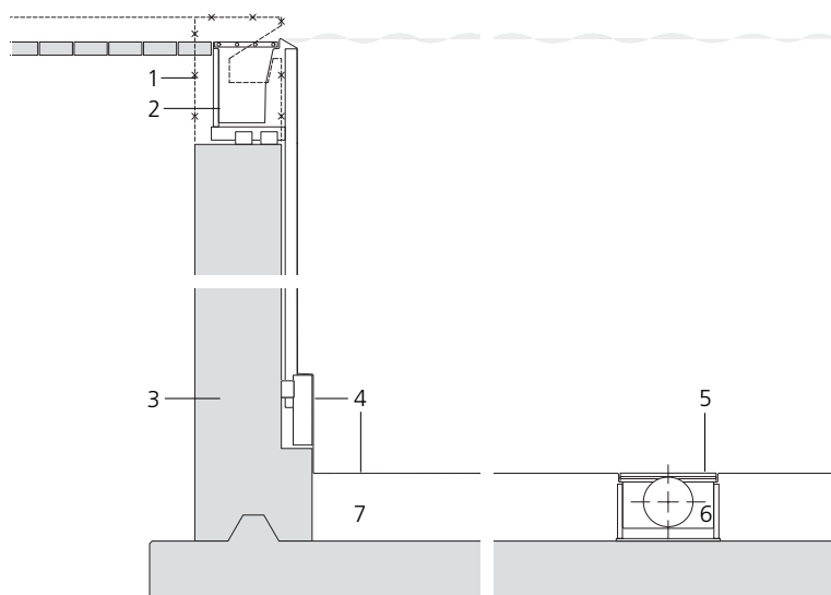
Schemaschnitt Maßstab 1:50
