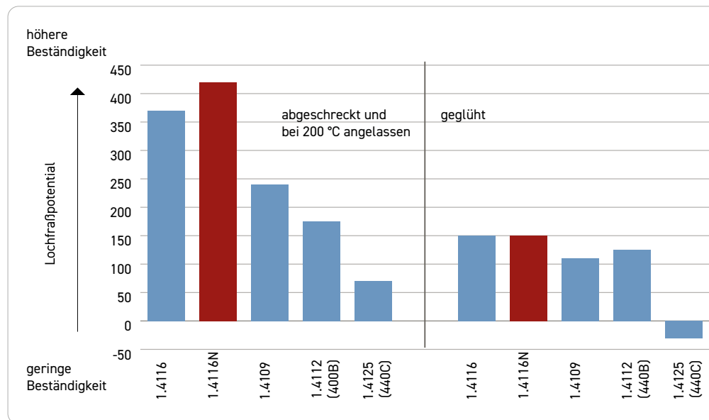
Abb. 2 Lochkorrosionsbeständigkeit in 0,02 M NaCl bei pH 6,6 und 23 °C (Quelle: Ugitech)
