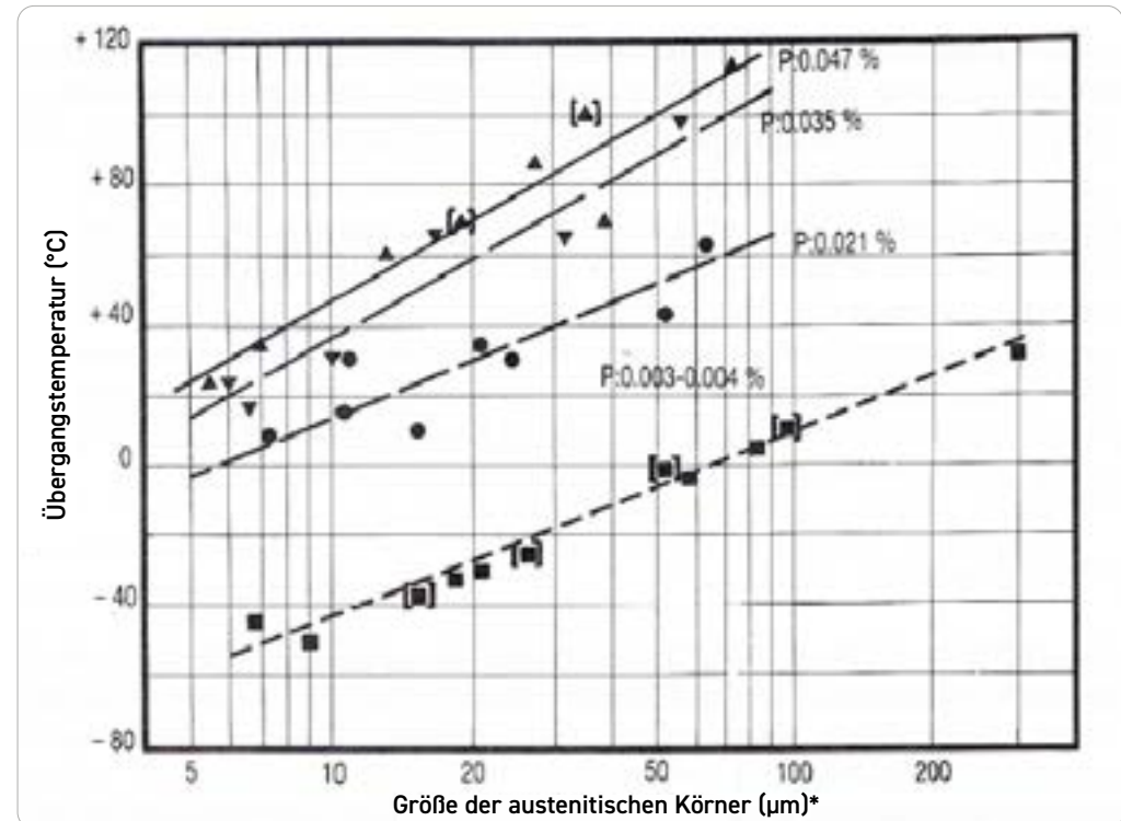
Abb. 5 Abhängigkeit der Übergangstemperatur von Rest-Phosphorgehalt und Korngröße bei einem martensitischen nichtrostenden Stahl mit 0,2 % C und 13 % Cr
